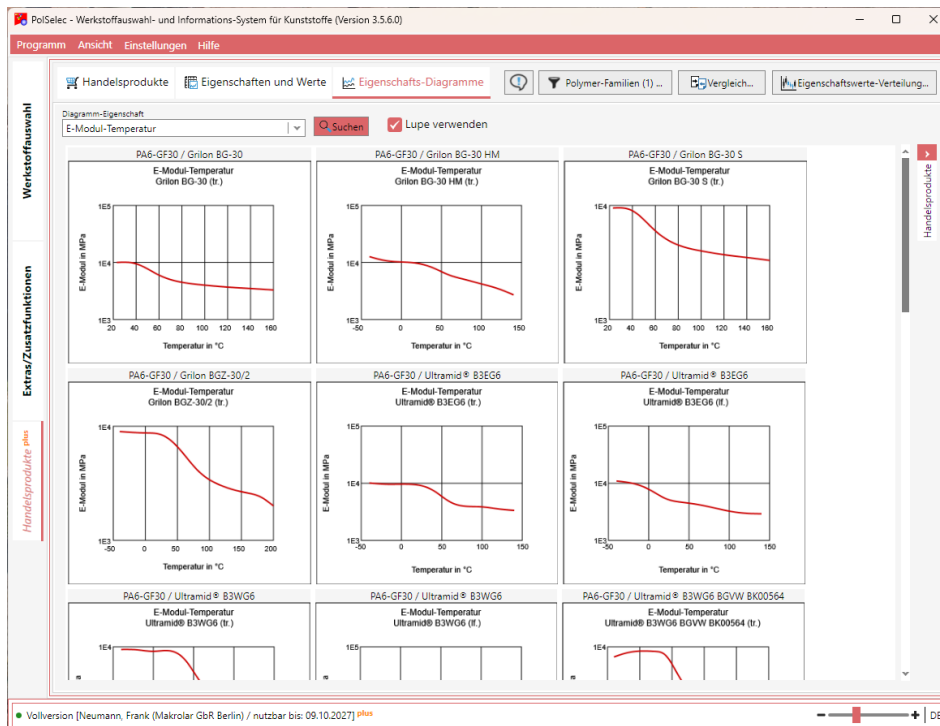
Abbildung 10: E-Modul-Temperatur-Diagramme für die Polymer-Familie PA6-GF30
